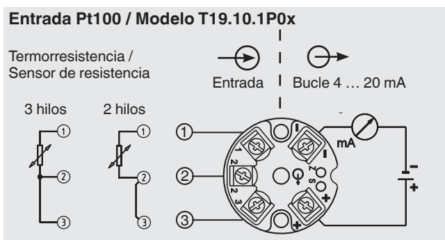
Transmisor modelo T19.10, versión cabezal
