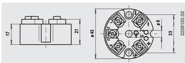
Transmisor modelo T19.10, versión cabezal
