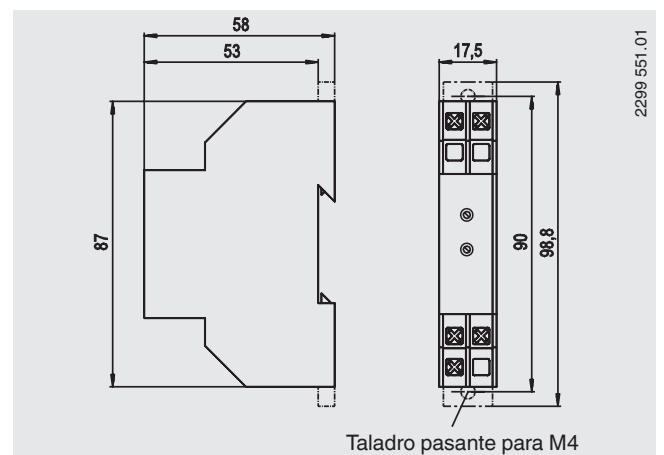
Transmisor modelo T19.30, versión de carril
