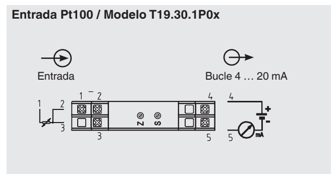
Transmisor modelo T19.30, versión de carril
