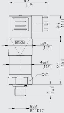
With angular connector DIN EN 175301-803 A
