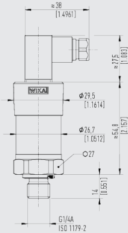
With angular connector DIN EN 175301-803 C
